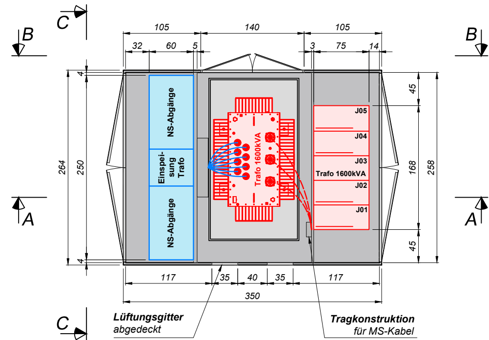
Grundriss
